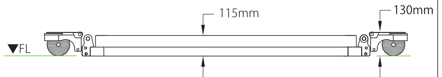
【モバイルモード断面図】
